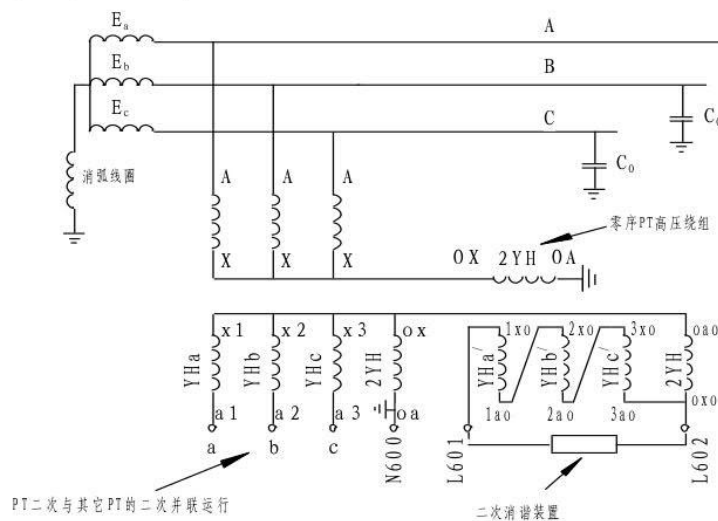
图九 4PT 接线方式三
