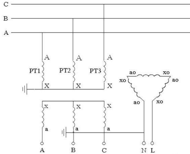
图五 B相接地方式
