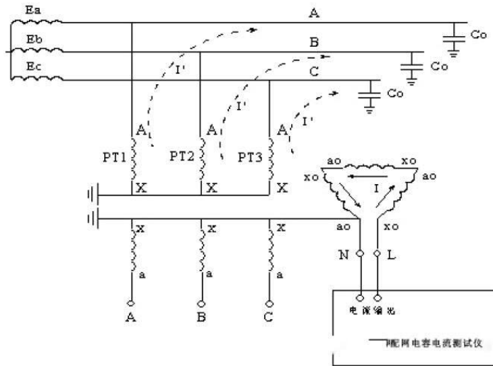
图二 测量原理图
