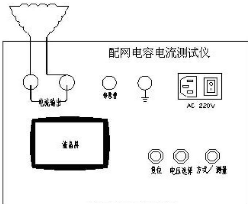
图十二 测量接线图
