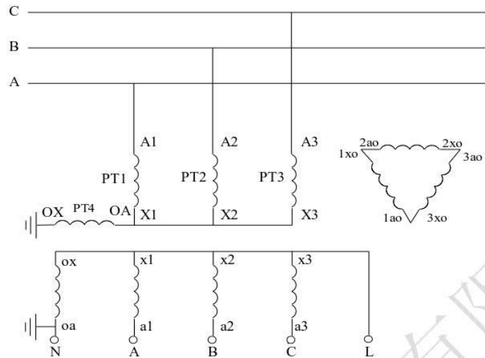
图七 4PT 接线方式一
