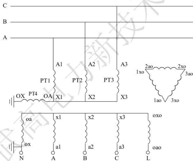
图八 4PT 接线方式二
