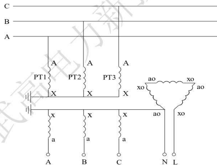
图四 N 接地方式
